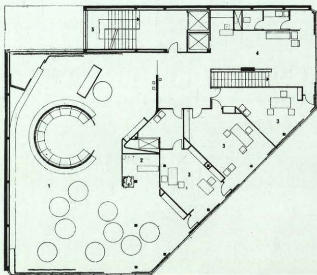
Planta zona dirección. Planta tipo.
